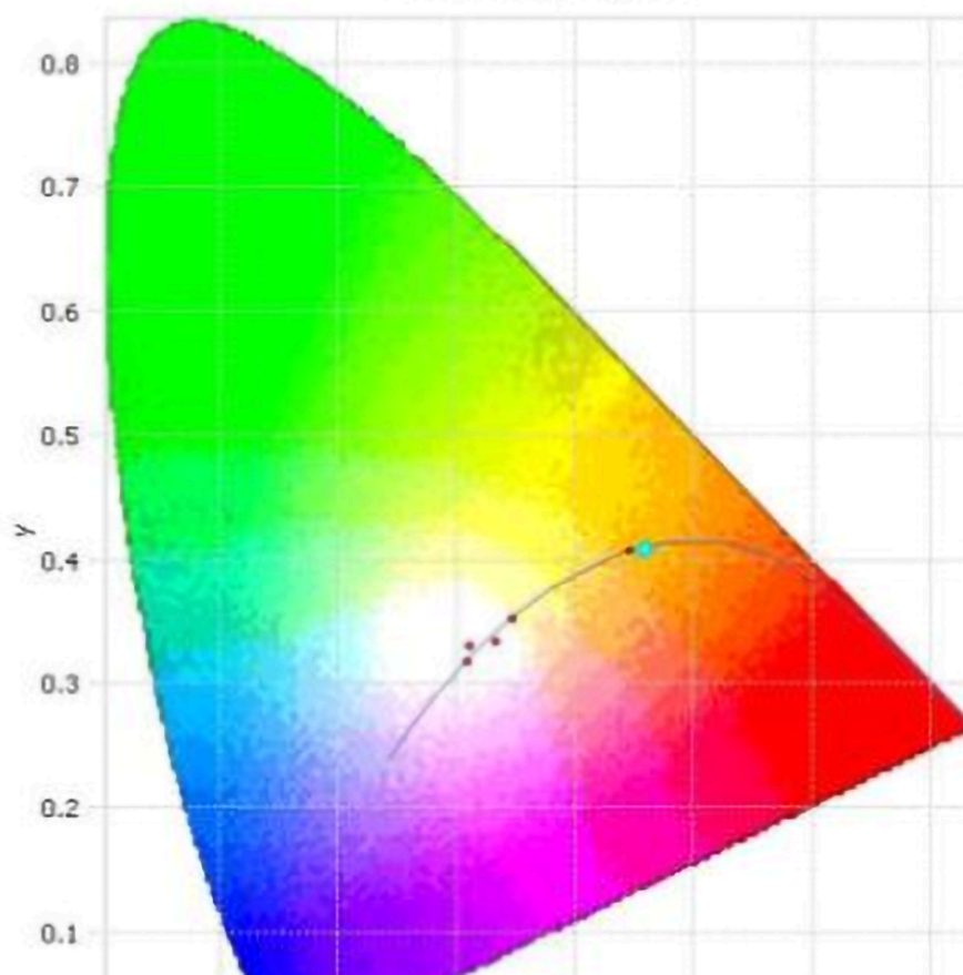
CIE 1931, 2 Degree
